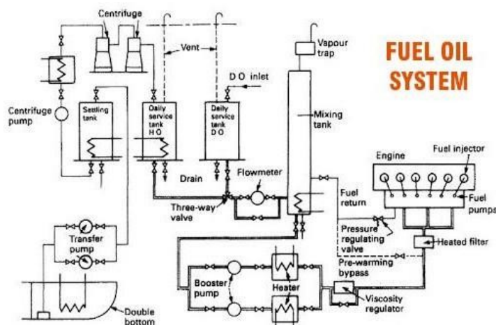
Gambar 2.9 Sistem bahan bakar
