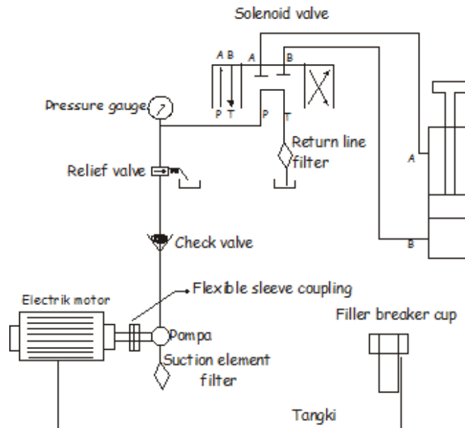
Gambar 2.3 Sistem LO hidroltik
